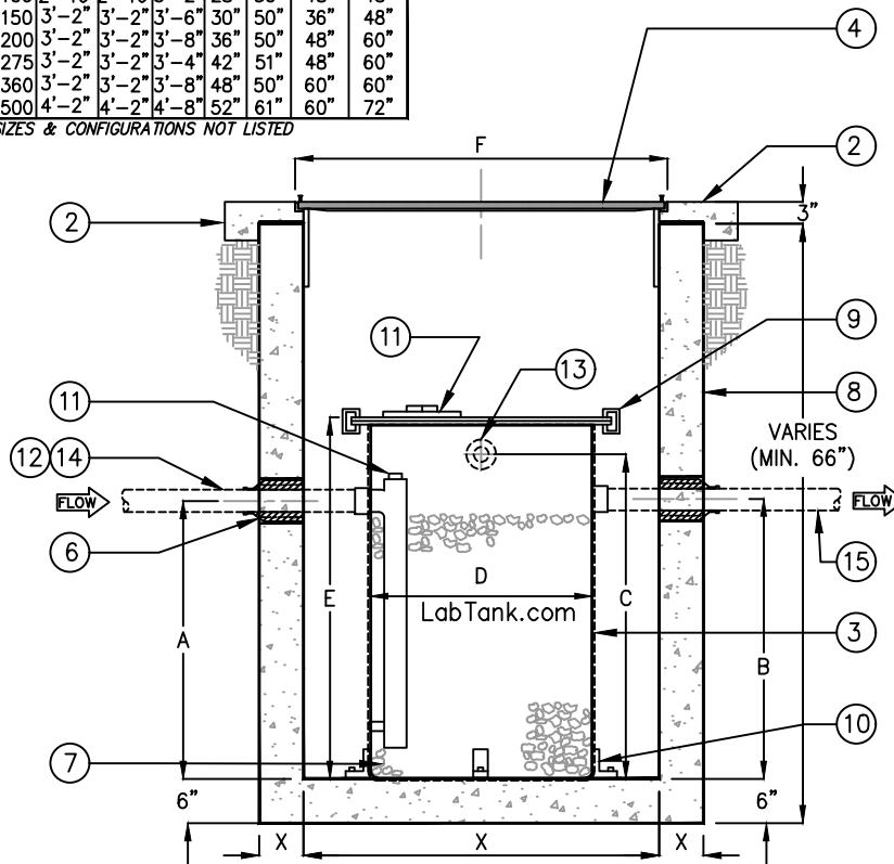
ELEVATION
